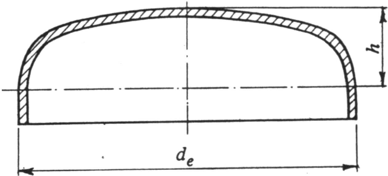
Черт.3. Заглушка эллиптическая
