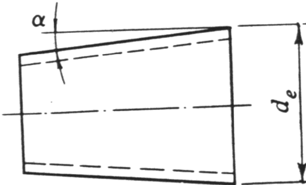
Черт.2. Концентрический переход
